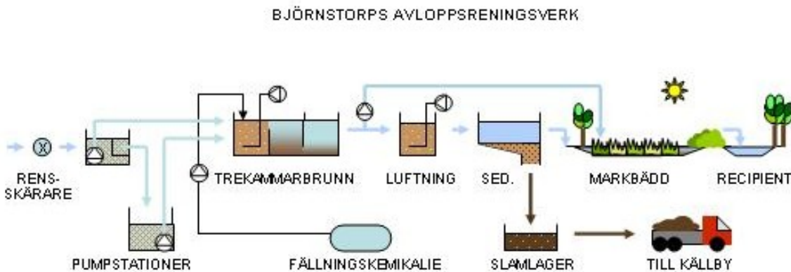
Figur 3. Principskiss över avloppsreningsverket i Björnstorp
